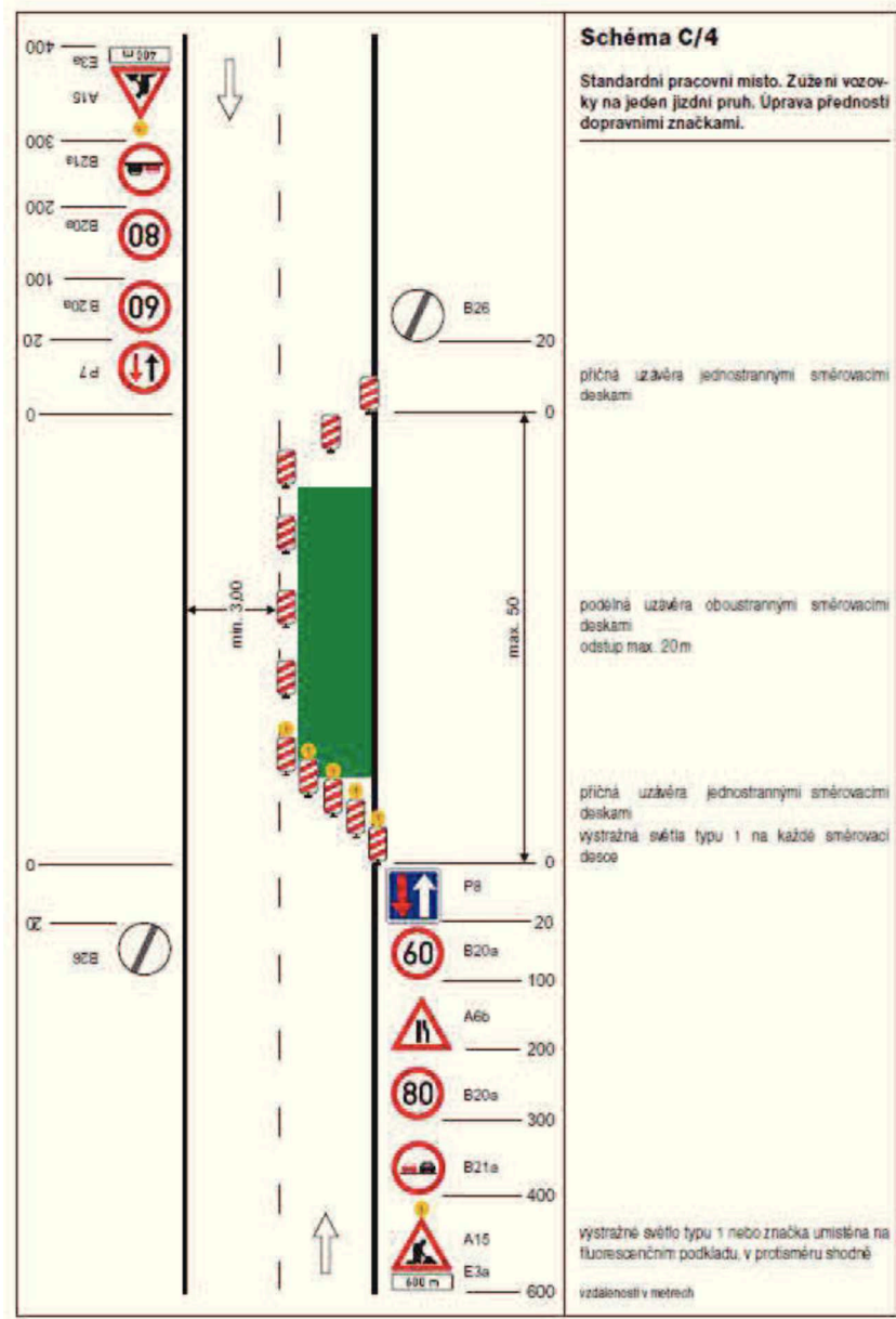
SCHÉMATA PRO OZNAČENÍ PRACOVNÍCH MÍST MIMO OBEC
