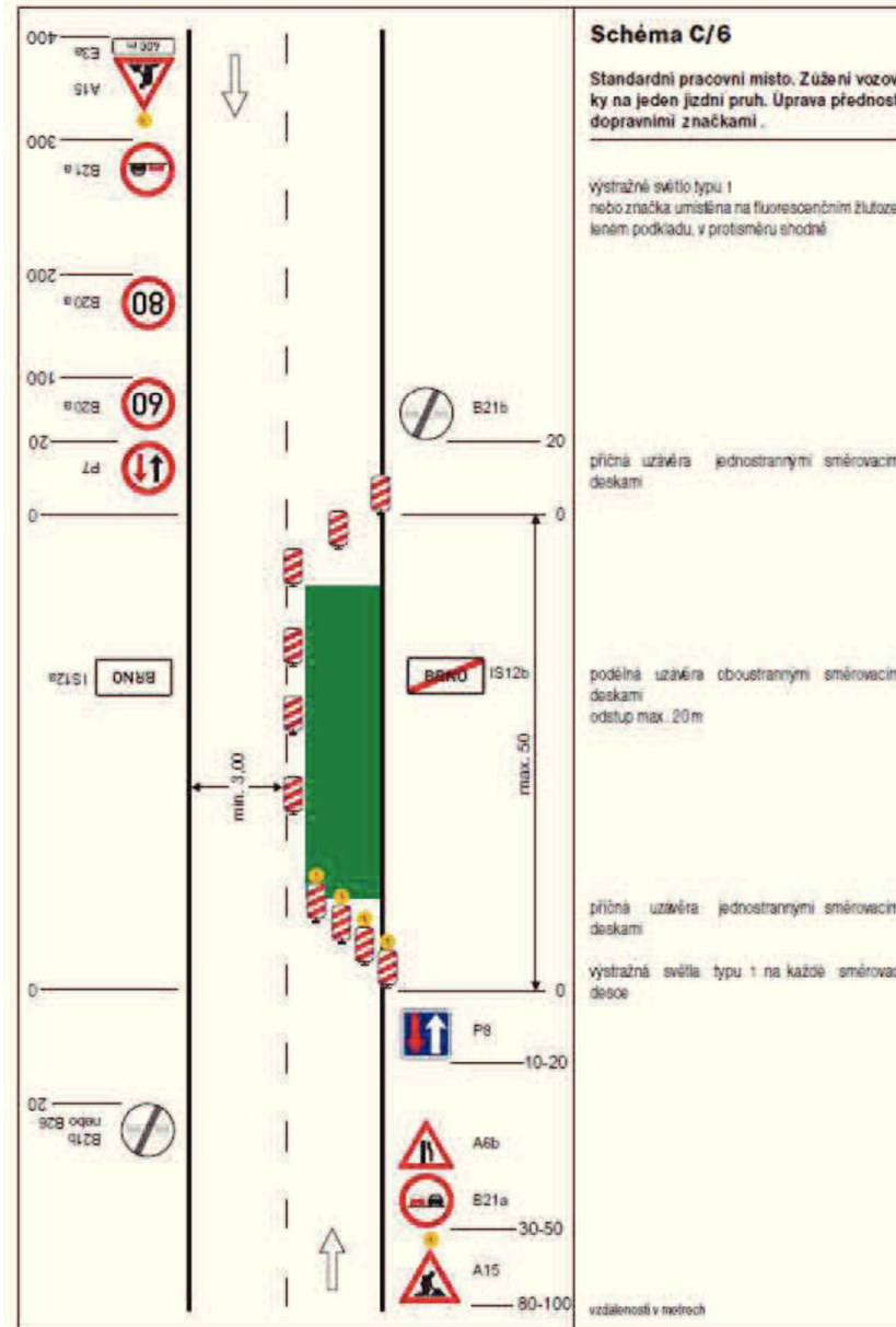
SCHÉMATA PRO OZNAČENÍ PRACOVNÍCH MÍST MIMO OBEČ
