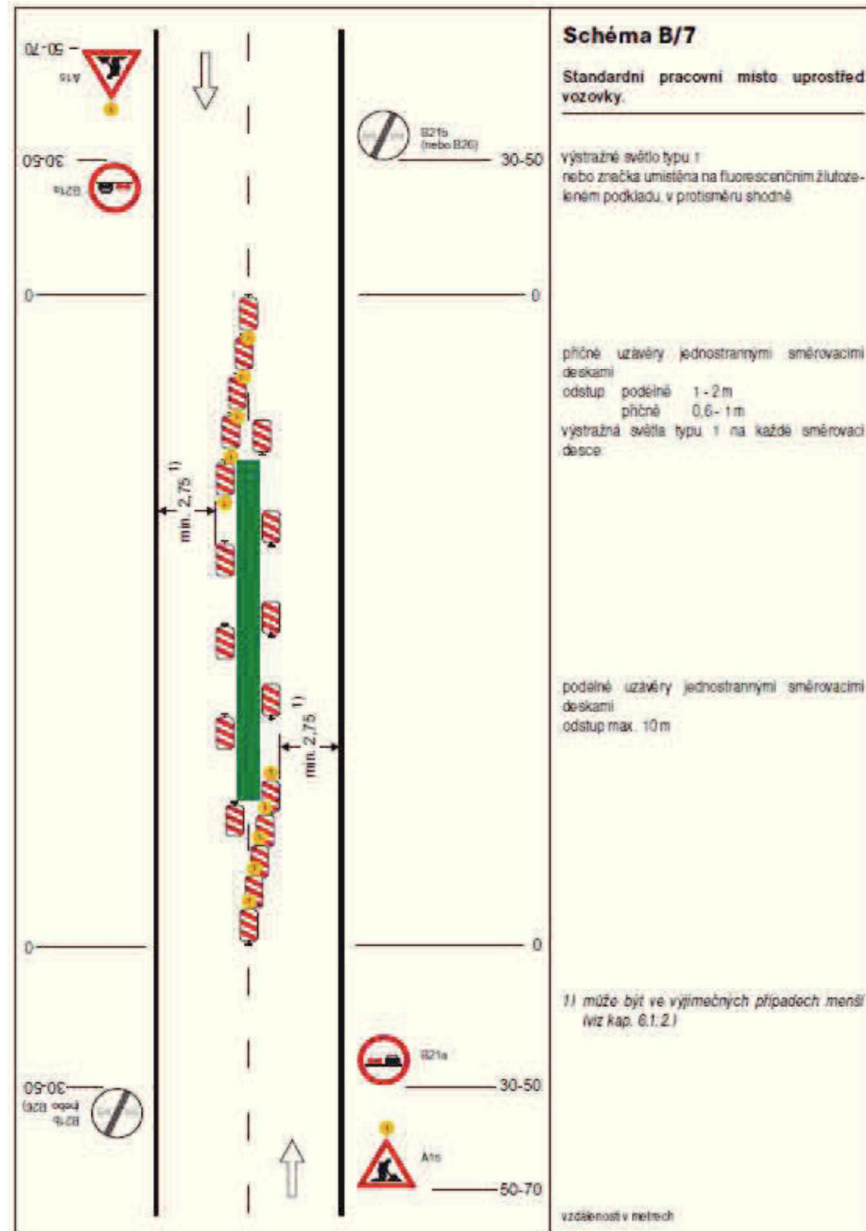
SCHEMATA PRO OZNACENÍ PRACOVNÍCH MÍST V OBCI
